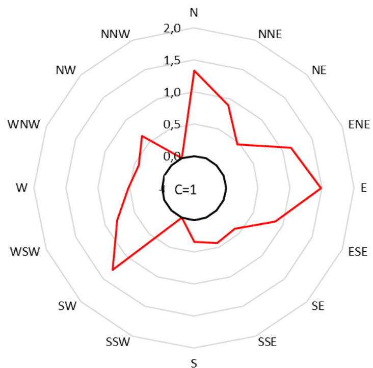
Slika 59 - Učestalost smjera vjetra [%] i srednje vrijednosti brzine vjetra [m/s] po smjerovima na mjernoj postaji 5-GOK natkriven određeni tijekom ljetnog razdoblja.
