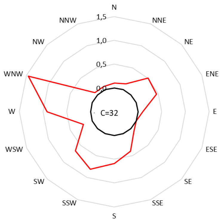
Slika 53 - Učestalost smjera vjetra [%] i srednje vrijednosti brzine vjetra [m/s] po smjerovima na mornoj postaji 4 – Mičevac određeni tijekom zimskog razdoblja.
