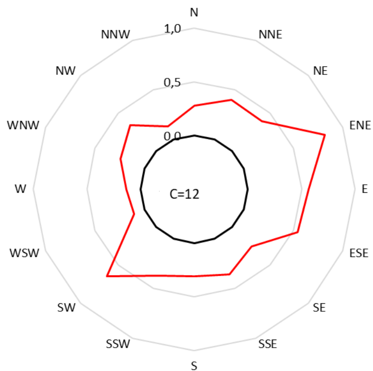
Slika 51 - Učestalost smjera vjetra [%] i srednje vrijednosti brzine vjetra [m/s] po smjerovima na mjernoj postaji 1 –Biologija sjever određeni tijekom jesenskog razdoblja.
