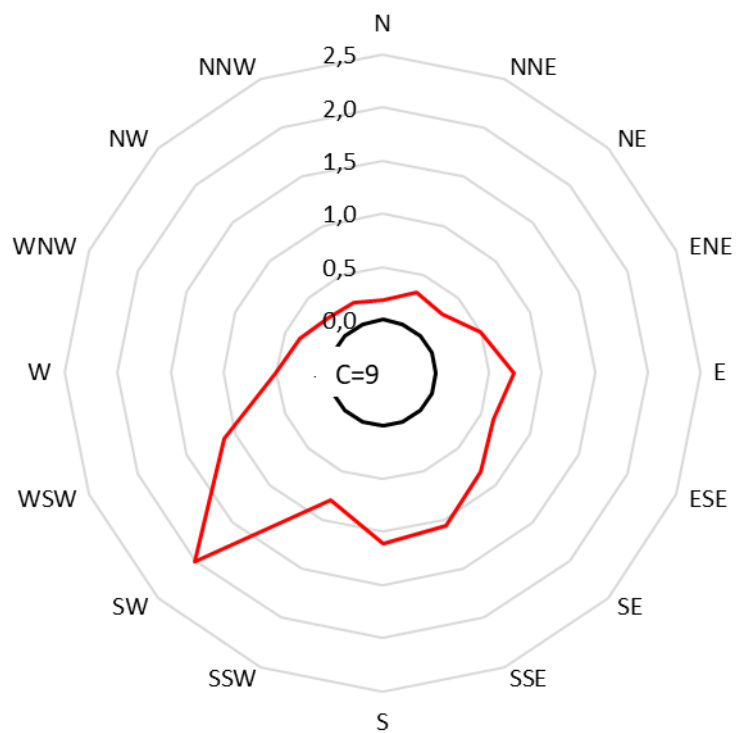
Slika 45 - Učestalost smjera vjetra [%] i srednje vrijednosti brzine vjetra [m/s] po smjerovima na mjernoj postaji 1 –Biologija sjever određeni tijekom zimskog razdoblja.
