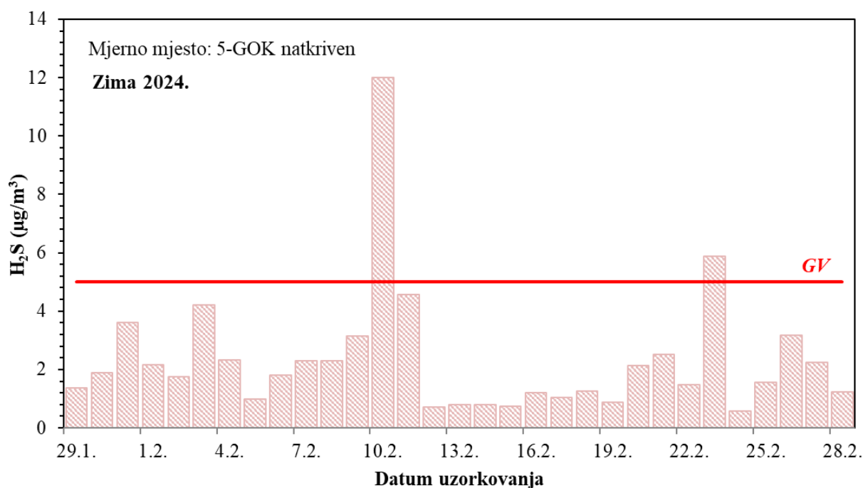
Slika 20 – Kretanje srednjih dnevnih koncentracija sumporovodika na mjestu 5 – GOK natkriven tijekom zimskog razdoblja mjerenja
