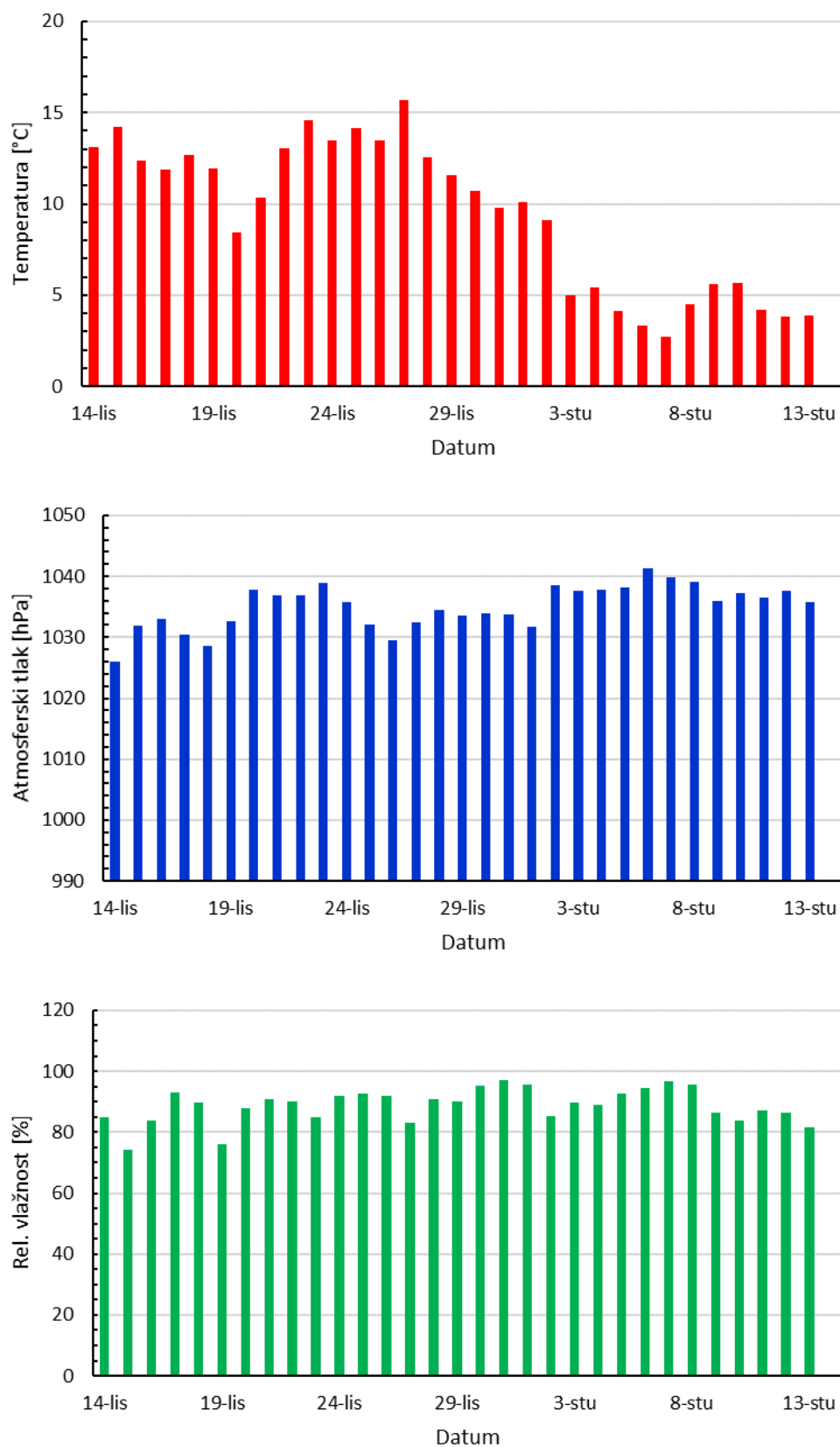
Slika 50 - Dnevni srednjaci temperature, tlaka i relativne vlažnosti na mjernoj postaji 1 –Biologija sjever određeni tijekom jesenskog razdoblja
