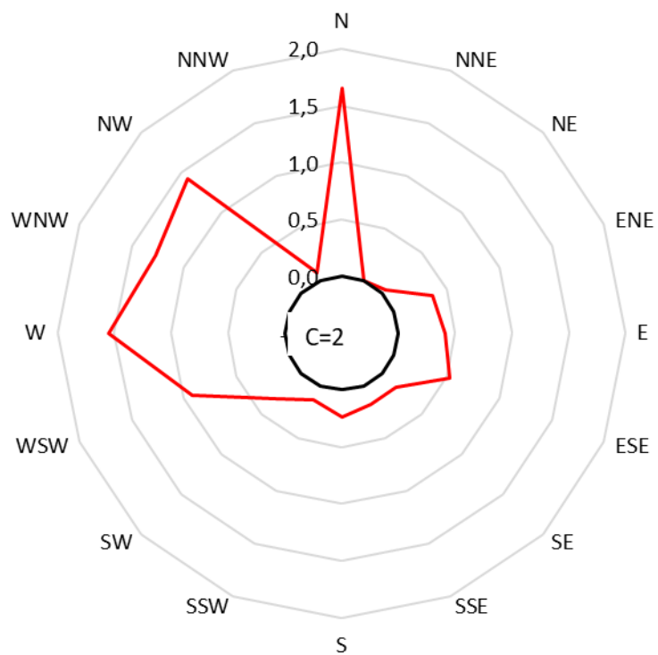
Slika 57 - Učestalost smjera vjetra [%] i srednje vrijednosti brzine vjetra [m/s] po smjerovima na mjernoj postaji 5-GOK natkriven određeni tijekom zimskog razdoblja.
