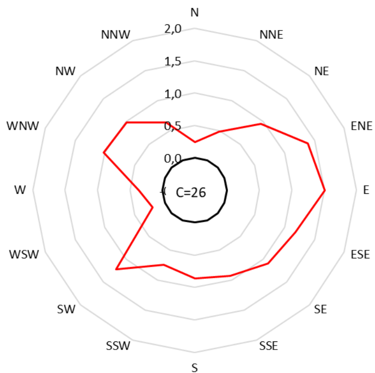
Slika 49 - Učestalost smjera vjetra [%] i srednje vrijednosti brzine vjetra [m/s] po smjerovima na mornoj postaji 1 –Biologija sjever određeni tijekom ljetnog razdoblja.
