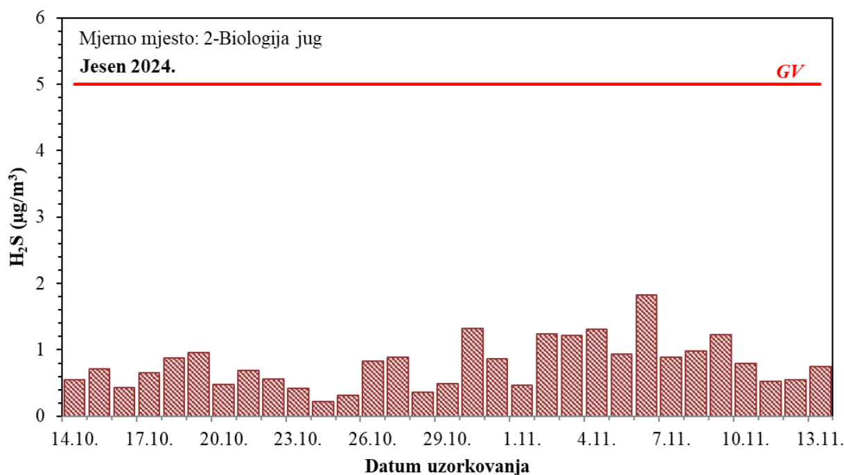
Slika 29 – Kretanje srednjih dnevnih koncentracija sumporovodika na mjernoj postaji 2 – Biologija jug tijekom jesenskog razdoblja mjerenja
