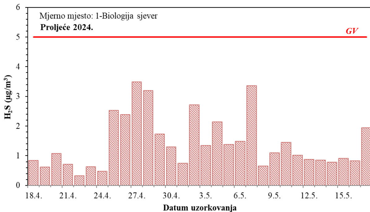
Slika 21 – Kretanje srednjih dnevnih koncentracija sumporovodika na mjestu 1 – Biologija sjever tijekom proljetnog razdoblja mjerenja
