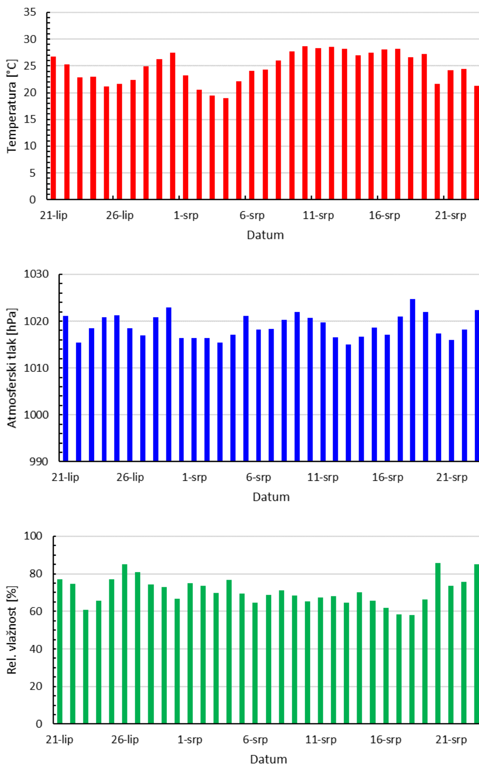
Slika 54 - Dnevni srednjaci temperature, tlaka i relativne vlažnosti na mjernoj postaji 4 - Mičevac određeni tijekom ljetnog razdoblja.
